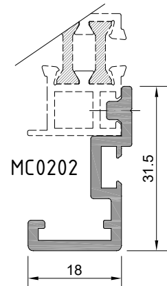
Profil No: MC0202 Ağırlık : 378 gr/m
