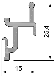
Profil No: SC0344 Ağırlık : 244 gr/m
